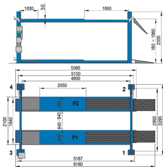
P4C 450 W CT - P4C 440 W L CT
